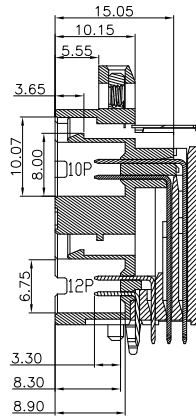
SECTION A-A
