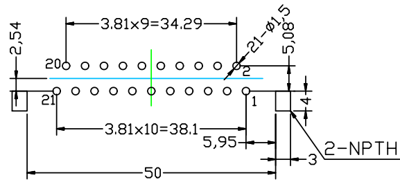
PCB HOLD PATTEN
